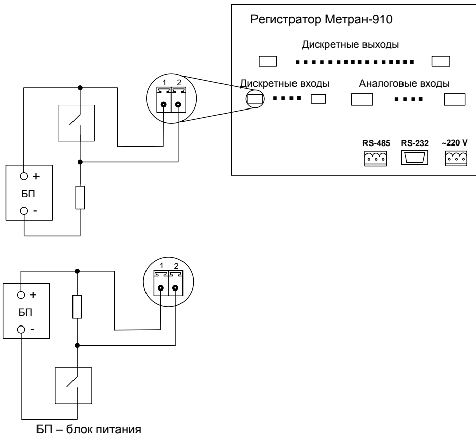
Рисунок В.7 – Схема подключения дискретных входов регистратора для потенциального подключения
