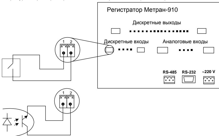
Рисунок В.4 – Схема подключения регистратора при измерении сопротивления (температуры термопреобразователем сопротивления) по 2-х проводной схеме
