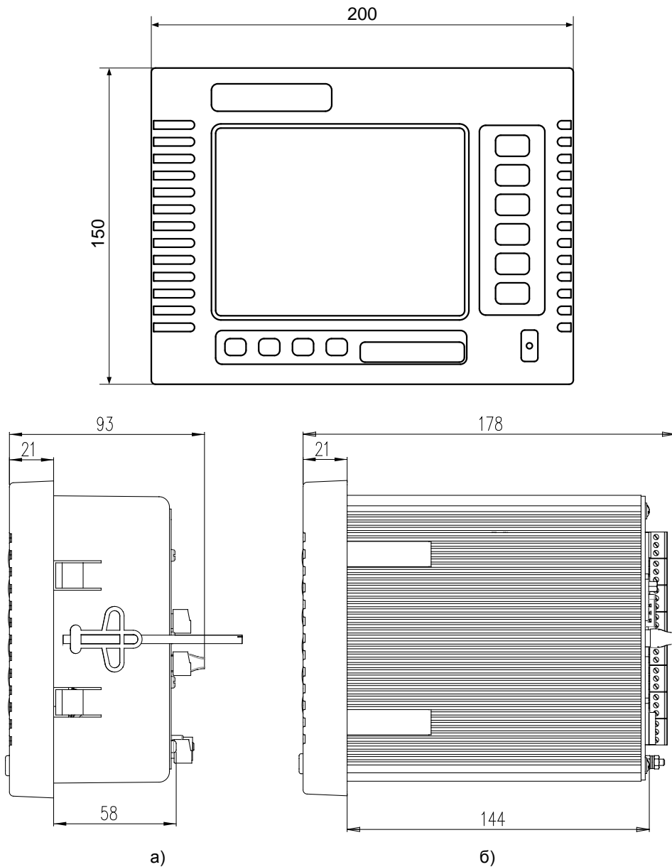
Рисунок А.1 – Габаритные размеры регистратора:
