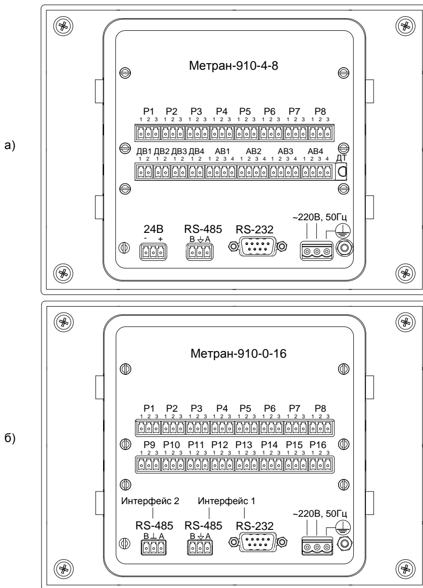
Рисунок Б.1 – Расположение разъемов на задней панели регистратора исполнения 1: а) для Метран-910-4-8, б) для Метран-910-0-16
